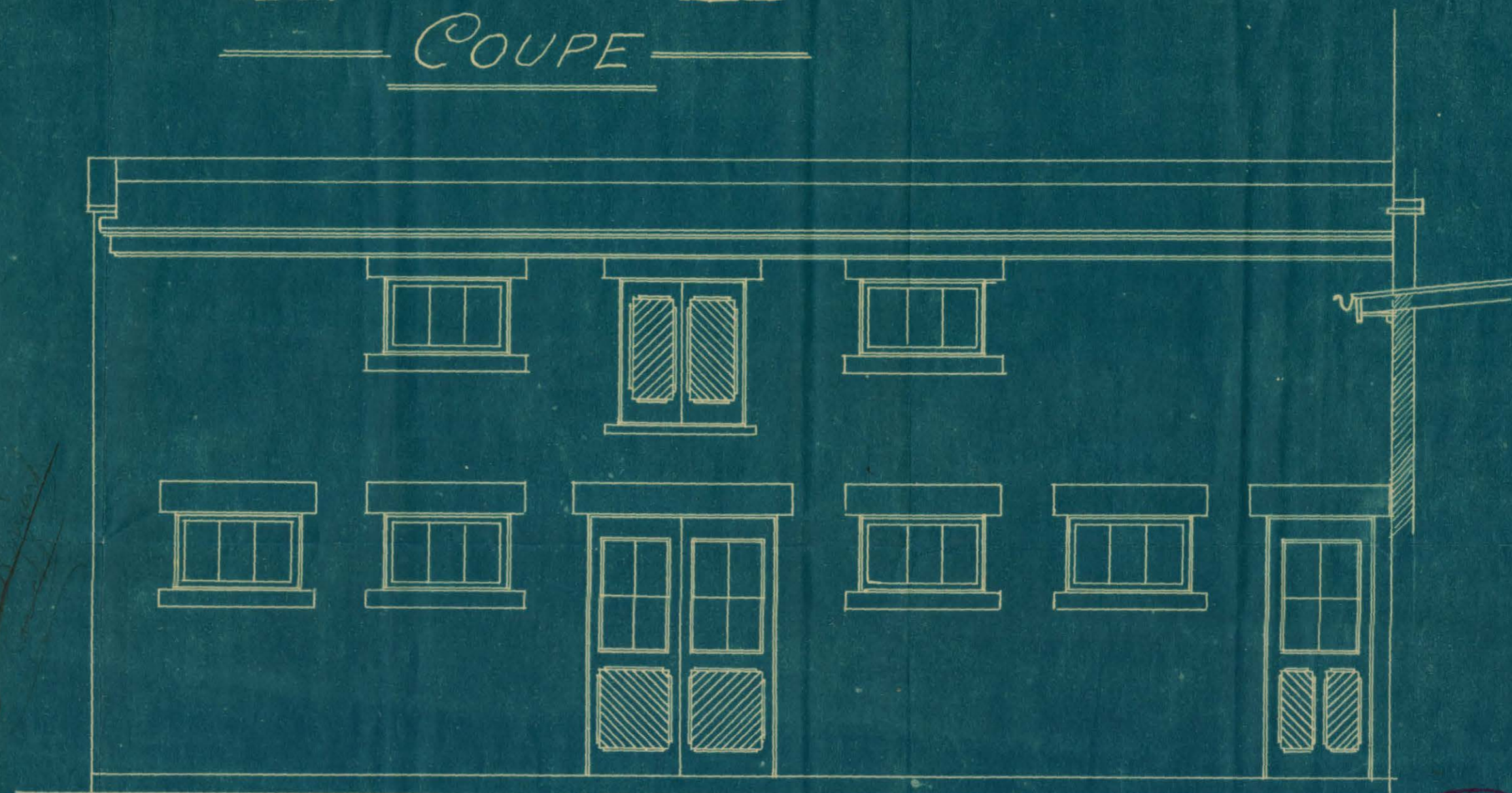
— ELEVATION —
