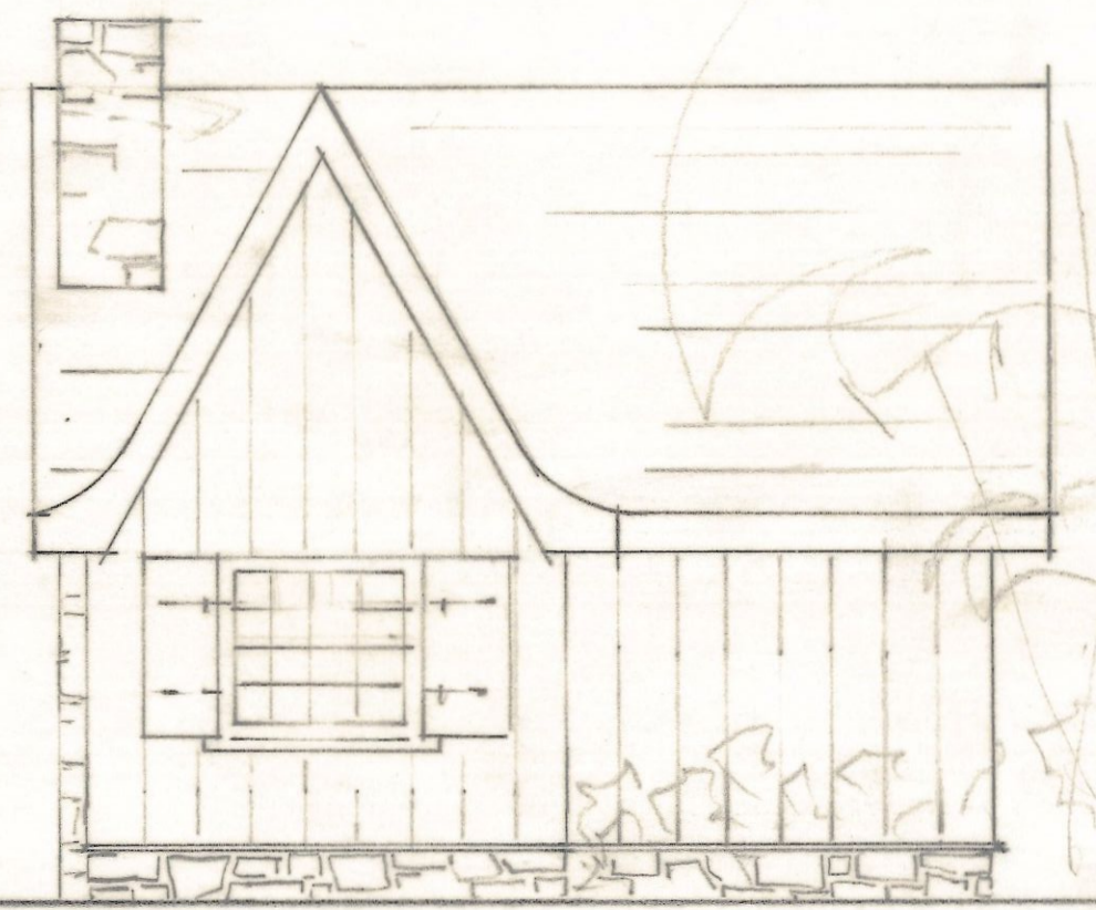
ELEVATION - 1
